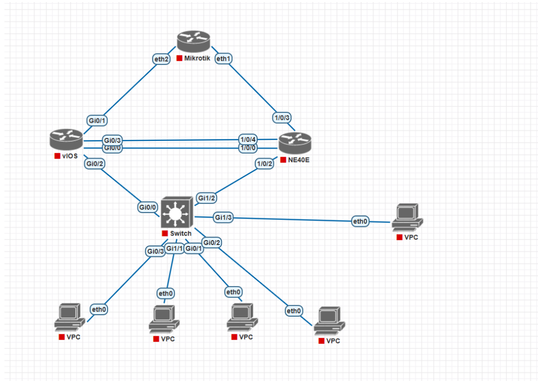
Gambar 2: Topologi Praktikum
