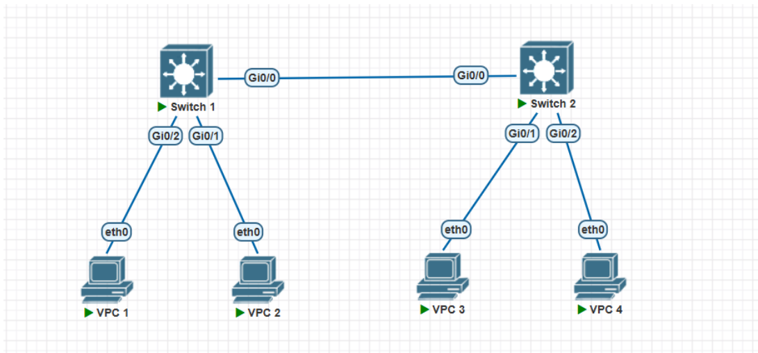
Gambar 1: Topologi Jaringan
